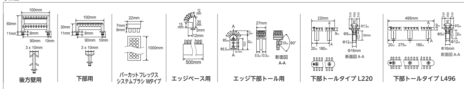
寸法図
